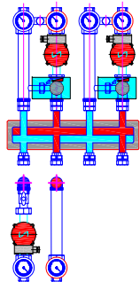
DOS CIRCUITOS MEZCLADO MAS CARGA DE TANQUE
